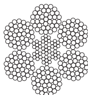
6x37M (18/12/6-1)+IWRC
