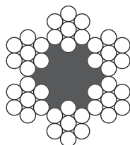
6х7 + Органический сердечник
