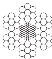
6x7 (6-1)+IWRC
