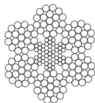
6x19M (12/6-1)+IWRC
