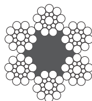
6x19S+ Органический сердечник
